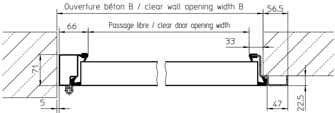
Profilé standard stock frame
