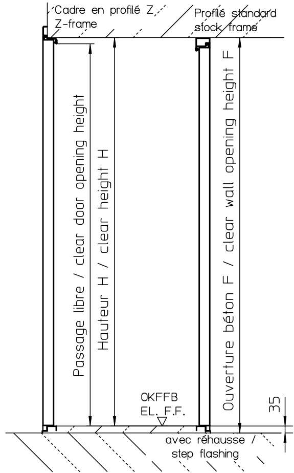
Cadre en profilé Z Z-frame
