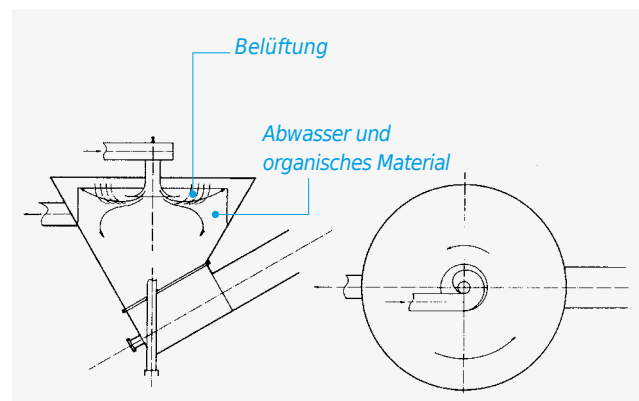
Prinzipische Skizze HUBER Coanda Sandklassierer RoSF3.
